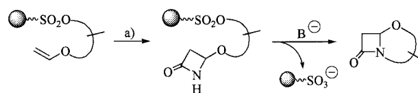
Scheme 1. a) i. CSI, Na 2 CO 3 ; ii. Red-Al
